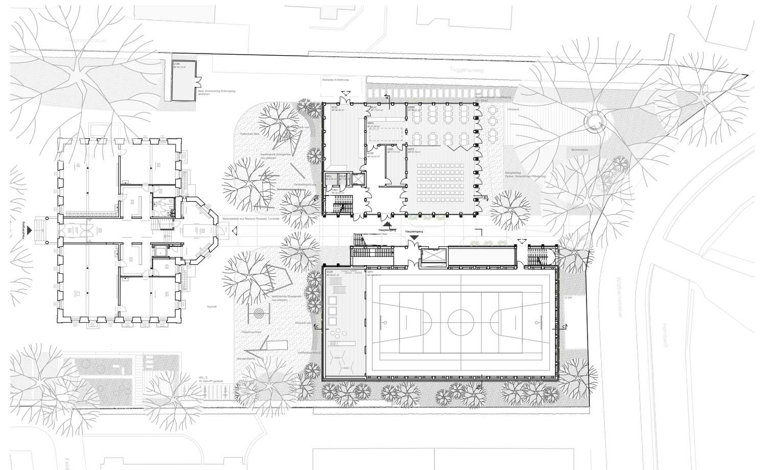
ERDGESCHOSS NEU
