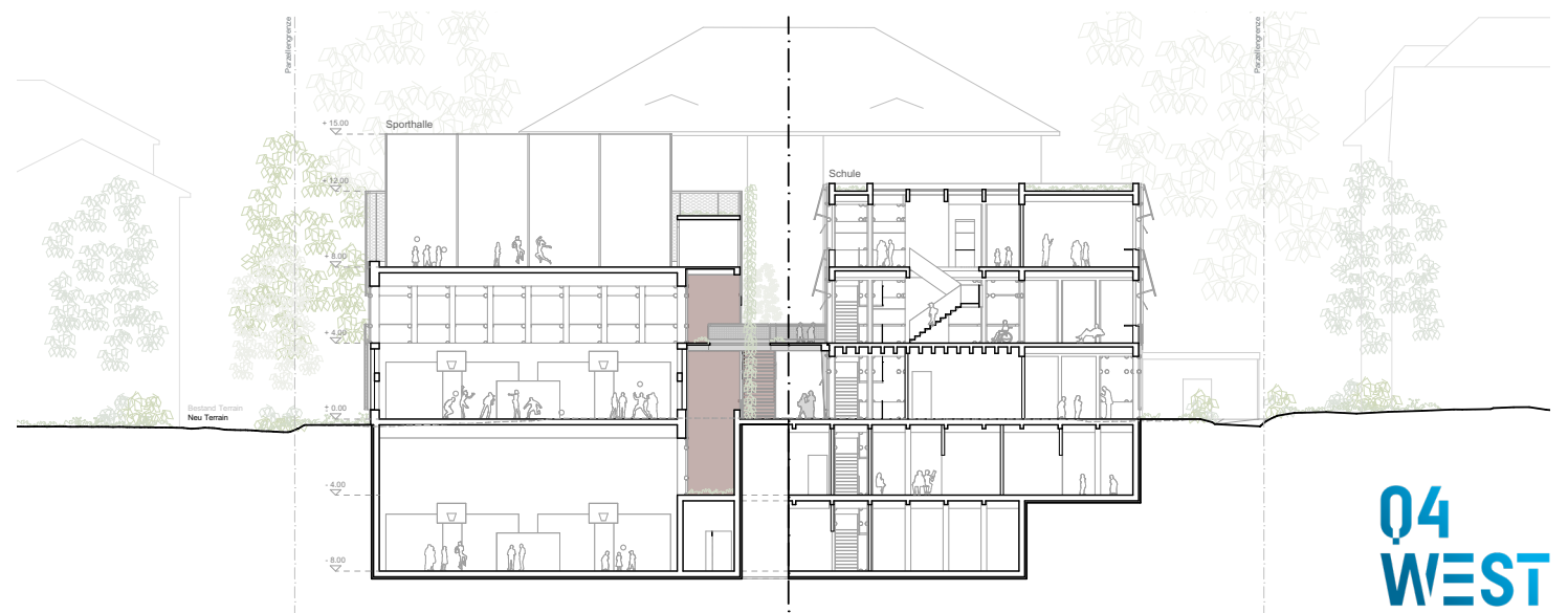
SCHNITT
